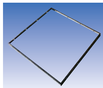
マンホールカバー砕 角型 サイズ：550×550㎜ 材質：SUS 304 厚み：2㎜
