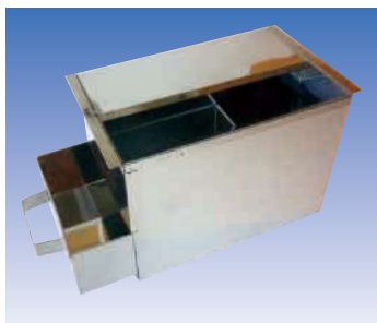
線香入れ サイズ：150×250×H175㎜ 材質：18-8ステンレス 厚み：1.0㎜
