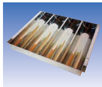
4連羊カントヨ サイズ：310×370×H50㎜ 材質：SUS 304 厚み：0.5㎜
